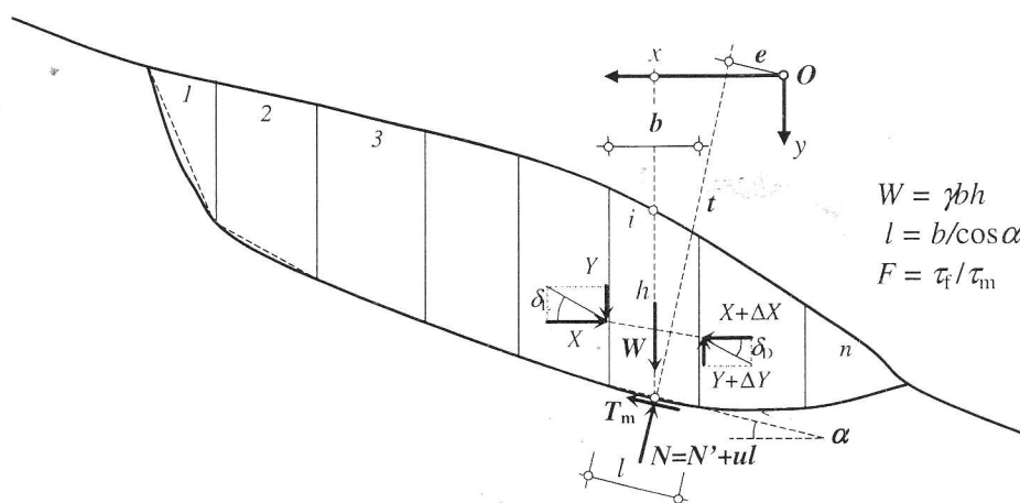
Slika 1. Geometrija, oznake i uticaji za jednu lamelu
